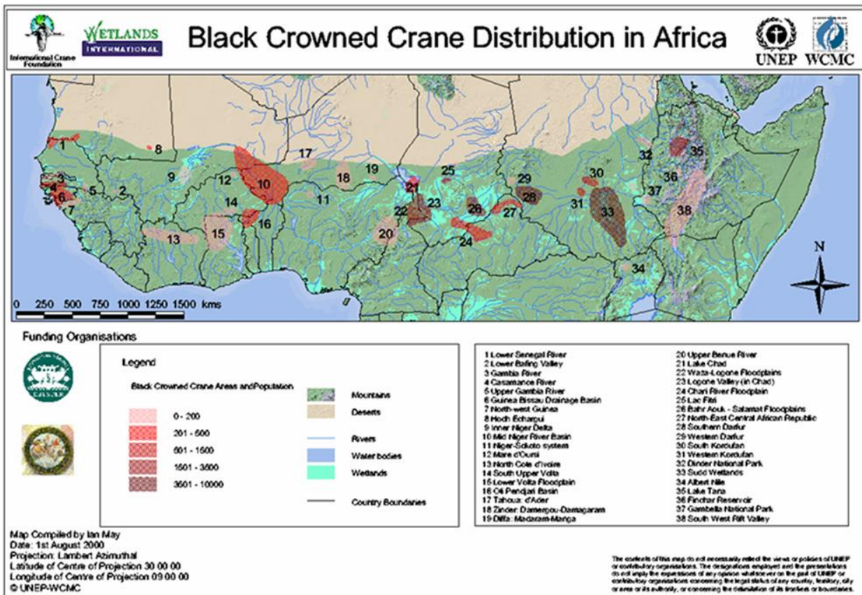
Figure 2 : Répartition de la Grue couronnée en Afrique (Williams & al., 2003)
